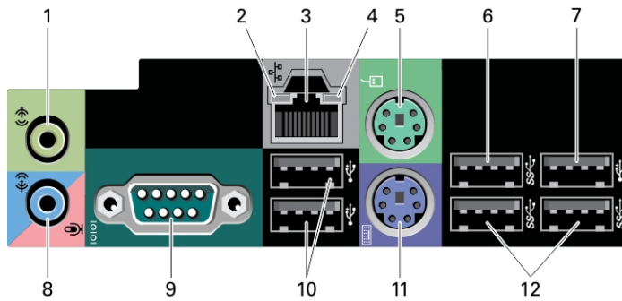
Figur 2. Bakpanelet til T3610/T5610
