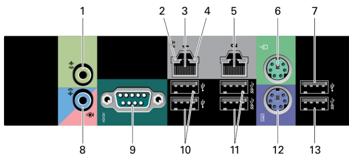
Figur 4. Oversikt over bakpanelet
