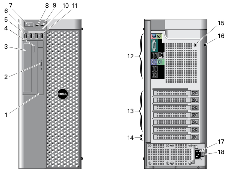
Figur 1. T3610/T5610 sett forfra og bakfra
